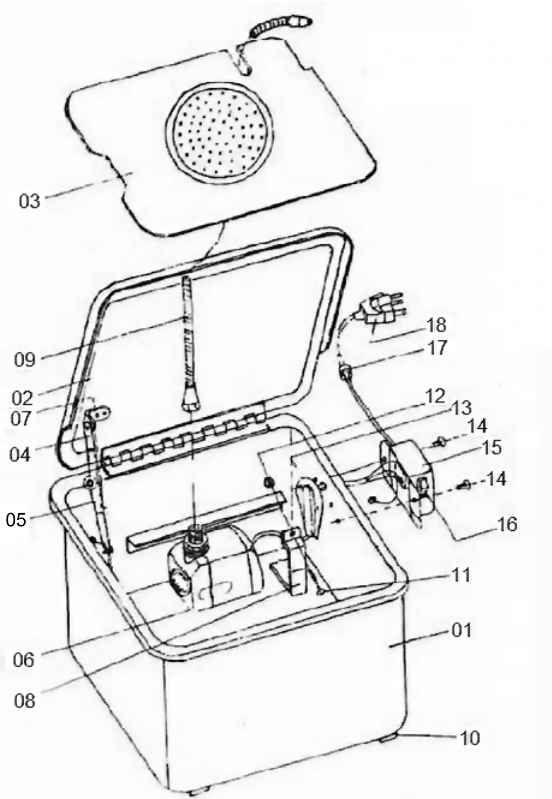
Abb. 13: Ersatzteilzeichnung TWG 20
