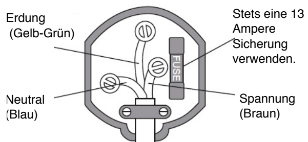
Abb. 10: Elektrischer Anschluss
