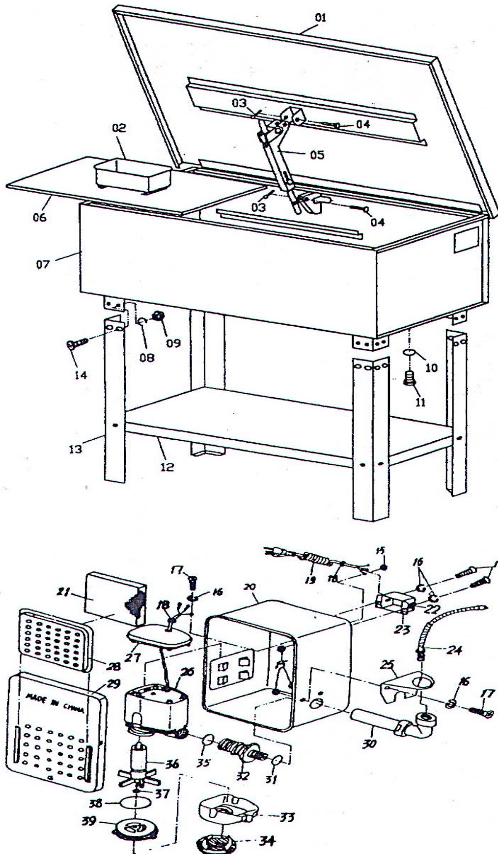
Abb. 15: Ersatzteilzeichnung TWG 150
