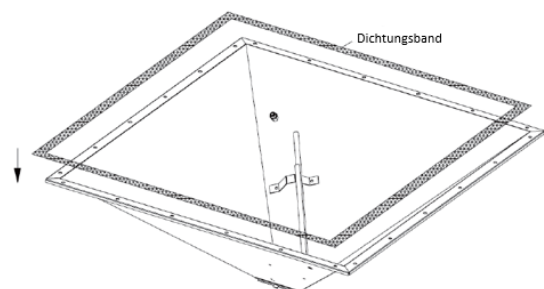
Abb. 5: Dichtungsband an der Unterseite des Rahmens
