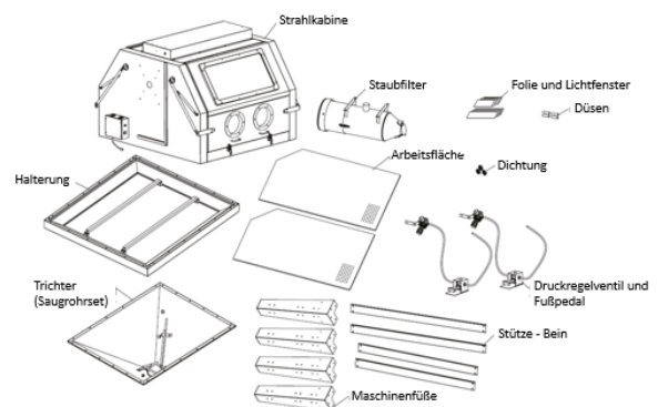
Abb. 4: Montageteile
