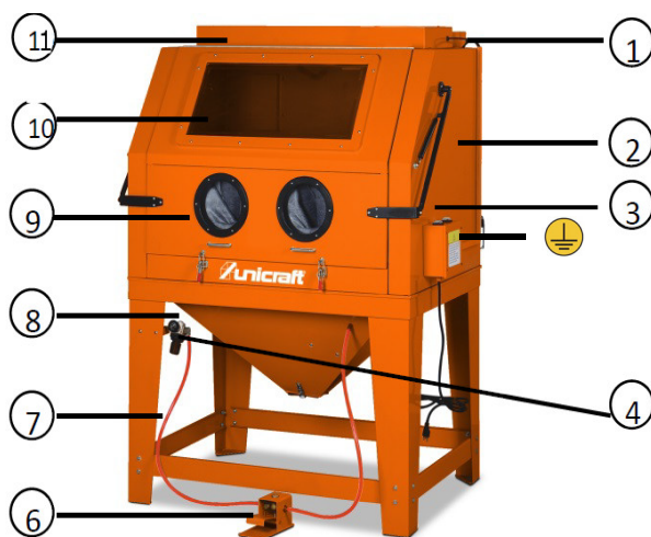
Abb. 3: Sandstrahlkabine SSK 5
