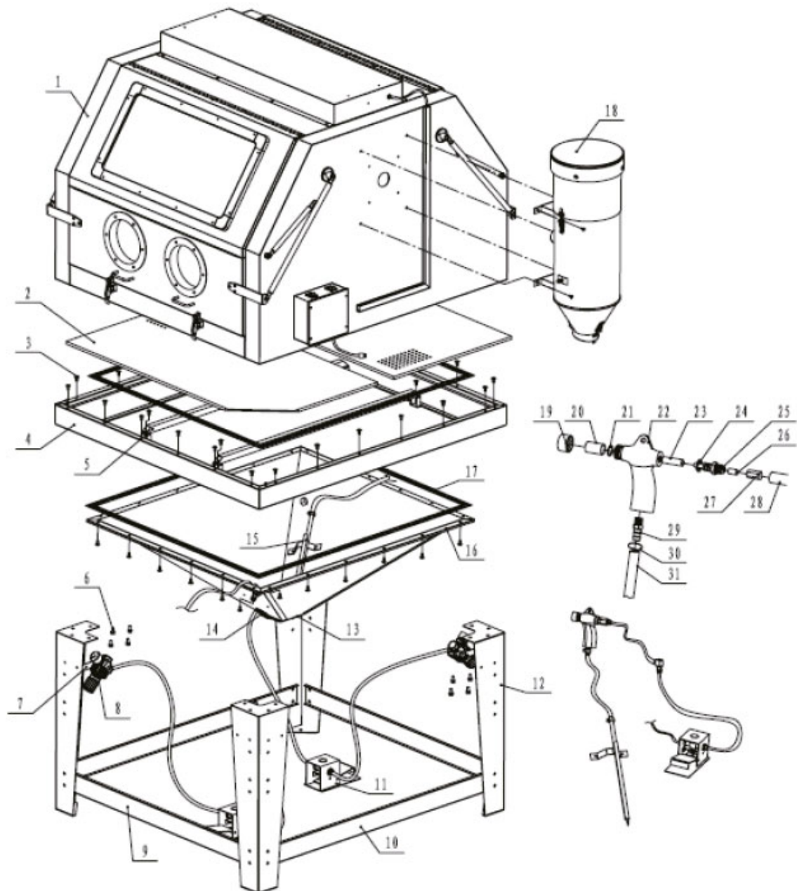
Abb. 16: Ersatzteilzeichnung 1 SSK 5
