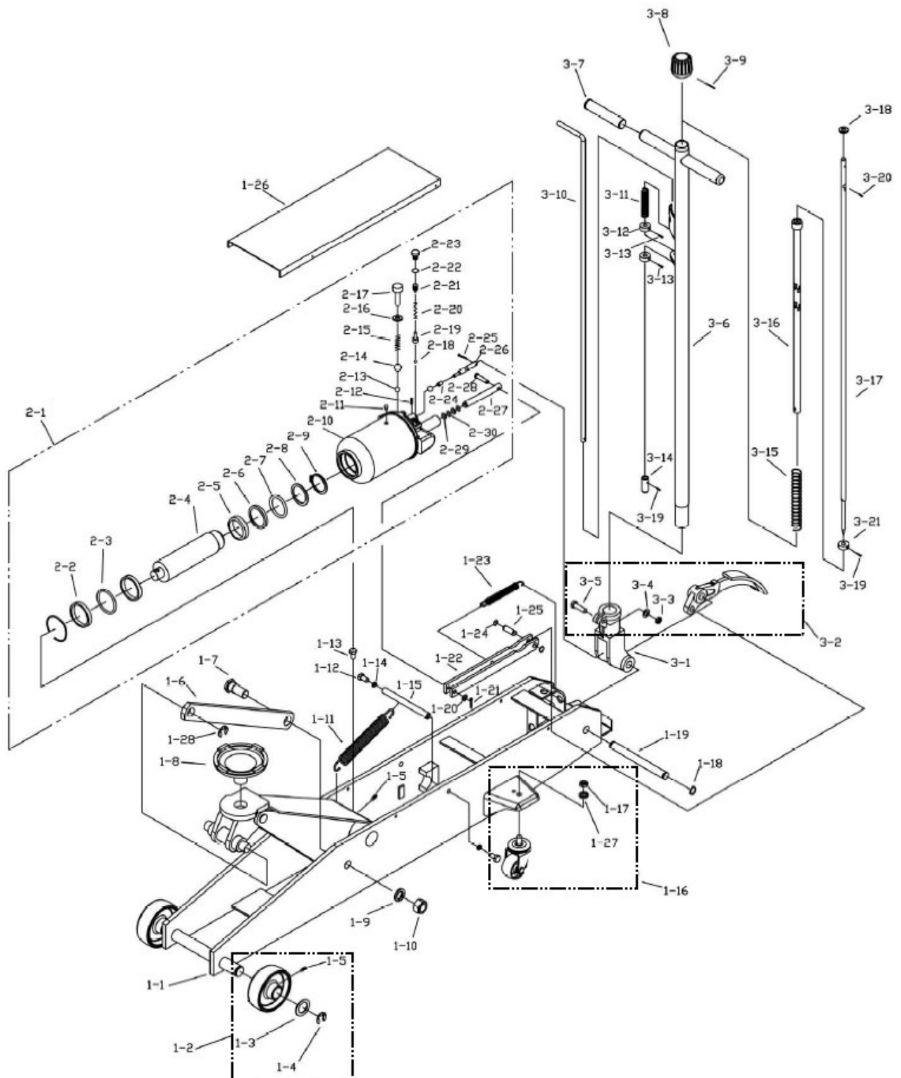
Abb. 9: Ersatzteilzeichnung 1
