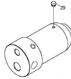
Abb. 9: Öleinfüllschraube
