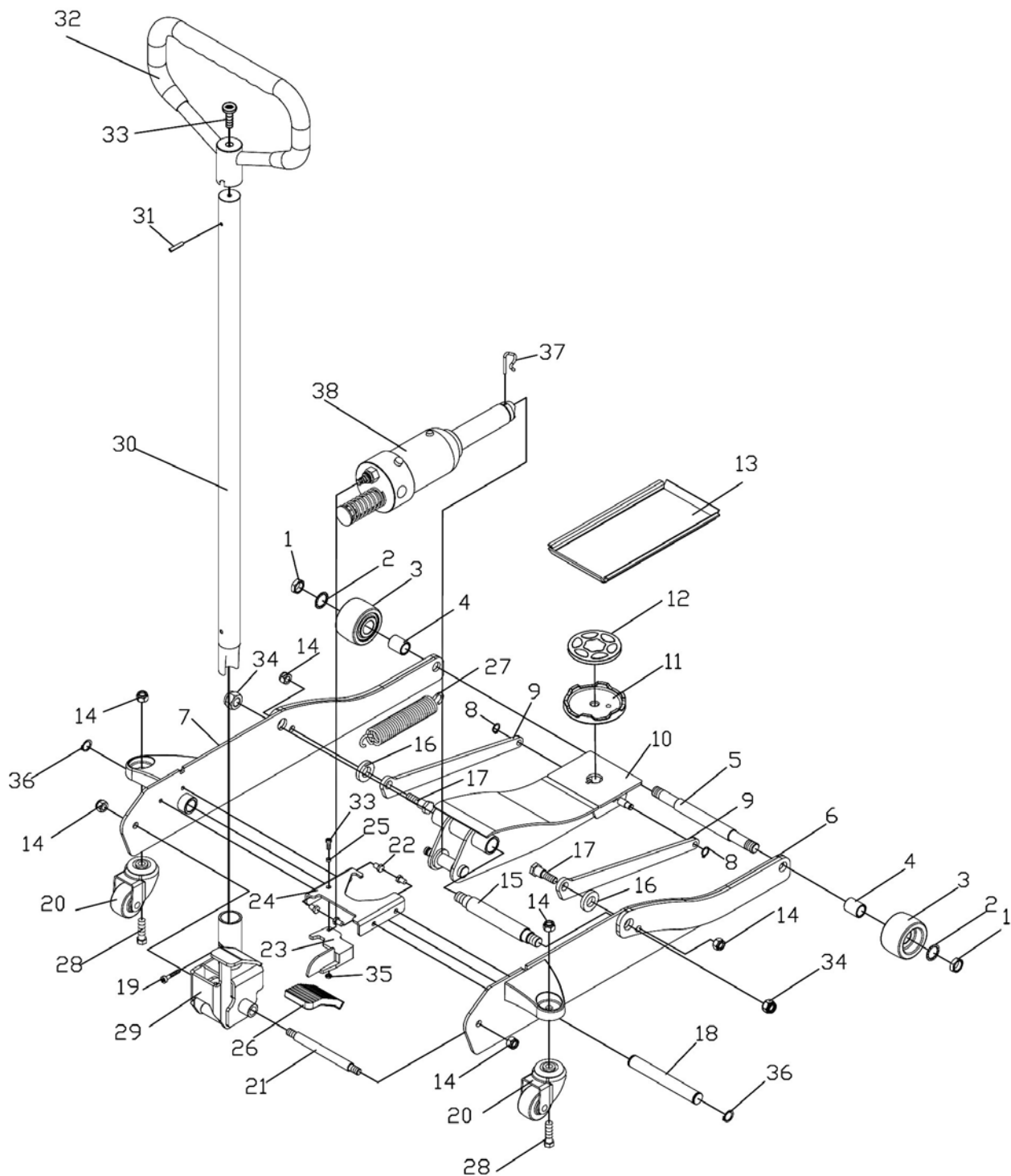
Abb. 10: Explosionszeichnung SRWH 2001 F
