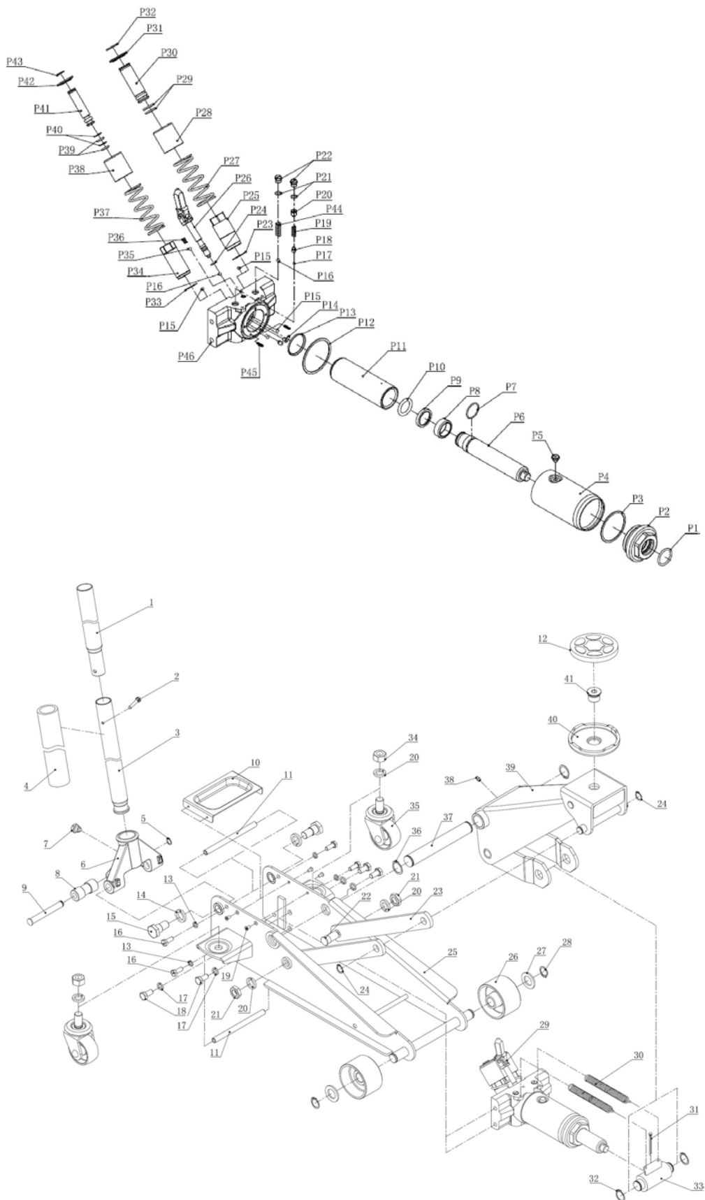
Abb. 14: Ersatzteilzeichnung 1 SRWH 3001 SIL
