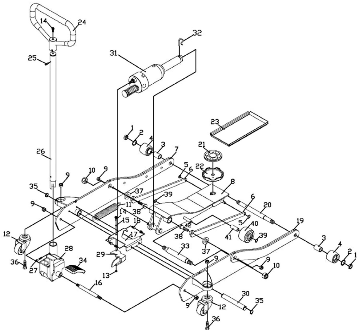
Abb. 11: Explosionszeichnung SRWH 2001 LF
