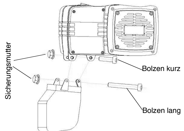
Abb. 6: Kettenbehälter befestigen
