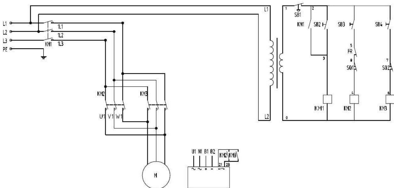
Abb. 13: Schaltplan EKZT-Modelle mit einer Hubgeschwindigkeit
