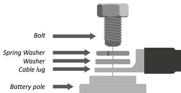
Batteriekabelverbindung
