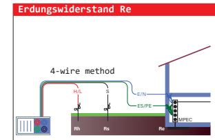
Abb. 17: Anschlussbild Erdungswiderstand (R E ), 4-Leiter
