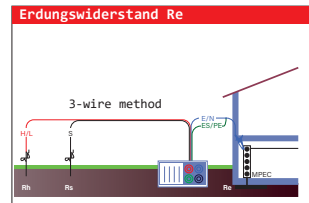
Abb. 16: Anschlussbild Erdungswiderstand (R E ), 3-Leiter
