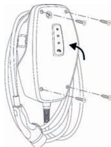
Fig. 16 : Fermeture du produit (exemple)
