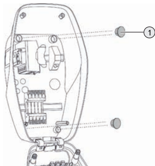
Fig. 7: Tappo (esempio)
