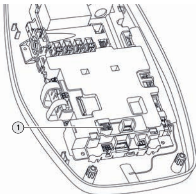
Fig. 12 : Prise Ethernet
