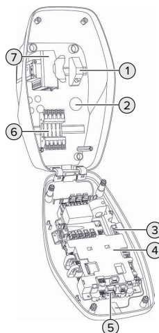
Afb. 3: Binnenaanzicht (voorbeeld)
