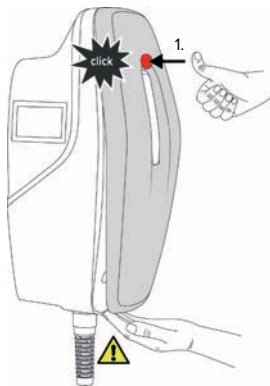
Afb. 18: Frontcover aanbrengen (voorbeeld) - 1
