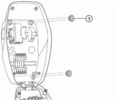
Fig. 7: Tapones de cierre (ejemplo)
