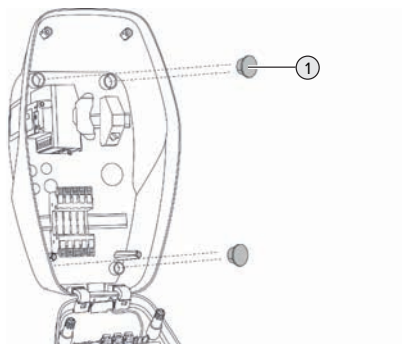
Abb. 7: Verschlussstopfen (Beispiel)
