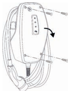
Afb. 5: Product openen (voorbeeld)
