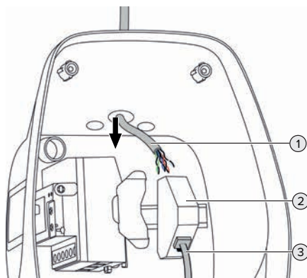
Fig. 13 : Branchement de la ligne de données (exemple)
