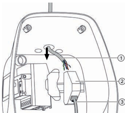
Fig. 13: Collegamento della linea di trasmissione dati (esempio)
