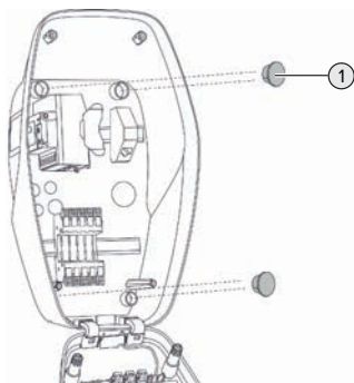
Afb. 7: Afsluitstoppen (voorbeeld)
