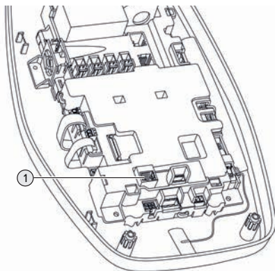
Fig. 12: Conexión Ethernet
