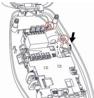
Afb. 14: Aansluiting downgrade-ingang
