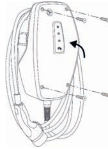
Fig. 16: Cerrar producto (ejemplo)
