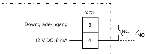
Afb. 15: Principeschema: aansluiting van een extern schakelcontact (standaardinstelling: NO)
