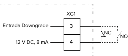
Fig. 15: Esquema de principio: Conexión de un contacto de conmutación externo (ajuste estándar: NC)
