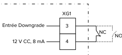
Fig. 15 : Schéma de principe : raccordement d'un contact électrique externe (réglage par défaut : NO)
