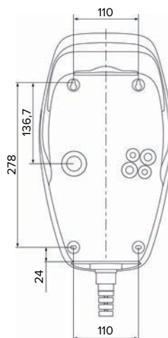
Fig. 6: Dimensiones de los taladros [mm]
