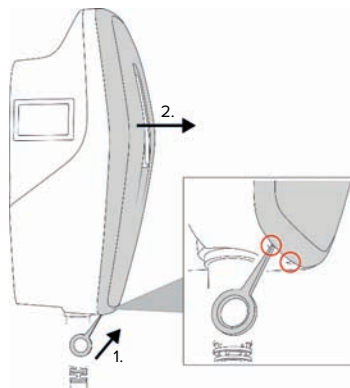
Fig. 4: Soltar la cubierta frontal (ejemplo)
