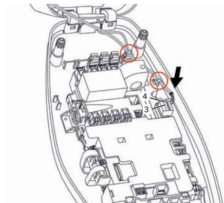
Abb. 14: Anschluss Downgrade-Eingang
