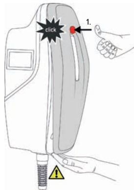
Abb. 18: Front Cover anbringen (Beispiel) - 1
