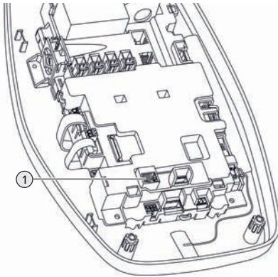
Abb. 12: Ethernet-Anschluss
