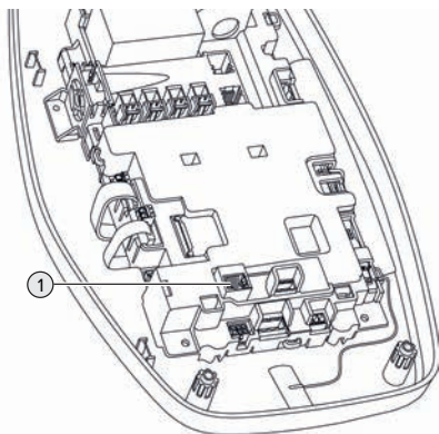
Afb. 12: Ethernetaansluiting
