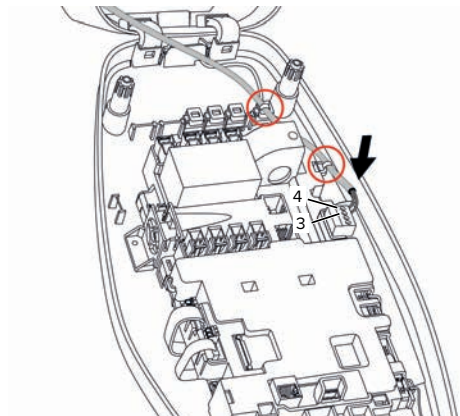
Abb. 14: Anschluss Downgrade-Eingang
