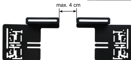
Figure 3 : Écart entre les supports de la caméra
