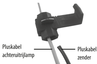
Afb. 4: Kabels plaatsen
