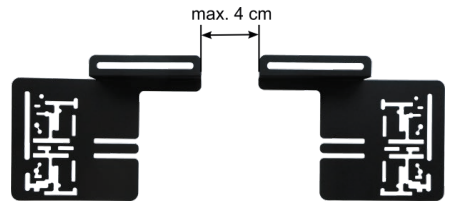
Bild 3: Abstand Kamerahalterungen
