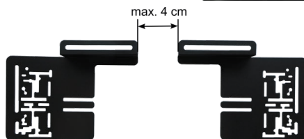
Afb. 3: Afstand camerahouders
