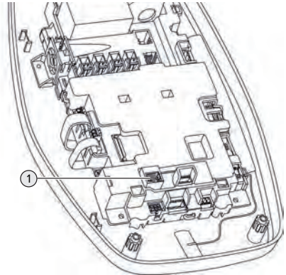
Afb. 13: Ethernetaansluiting
