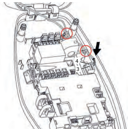
Abb. 15: Anschluss Downgrade-Eingang
