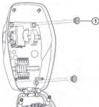
Afb. 7: Afsluitstoppen
