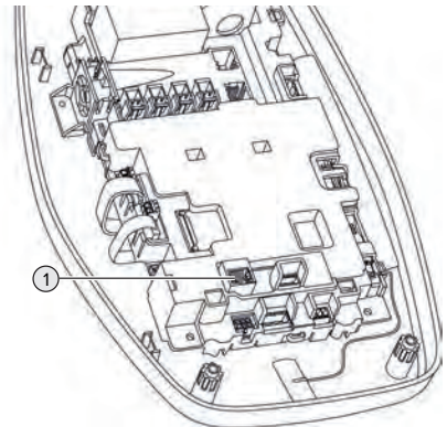
Abb. 13: Ethernet-Anschluss
