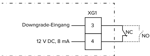
Abb. 16: Prinzipschaltbild: Anschluss eines externen Schaltkontakts (Standard-Einstellung: NO)
