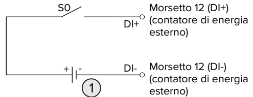
Fig. 17: Pilotaggio attraverso un relè di accoppiamento e un'alimentazione di tensione aggiuntiva (allo stato di consegna)
