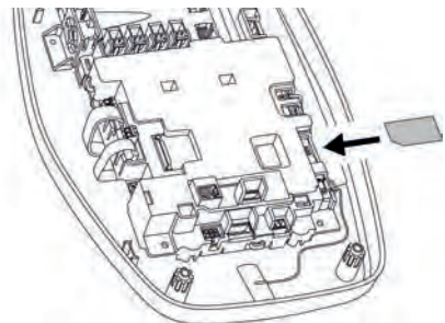
Afb. 11: SIM-kaart plaatsen
