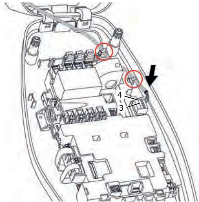
Afb. 15: Aansluiting downgrade-ingang
