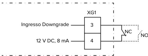
Fig. 16: Diagramma unifilare: collegamento di un contatto di commutazione esterno (impostazione di default: NO)
