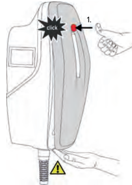
Fig. 20: Colocación de la cubierta frontal - 1
