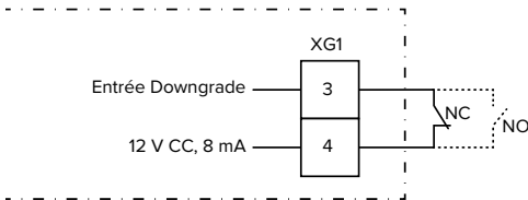
Fig. 16 : Schéma de principe : raccordement d'un contact électrique externe (réglage par défaut : NO)
