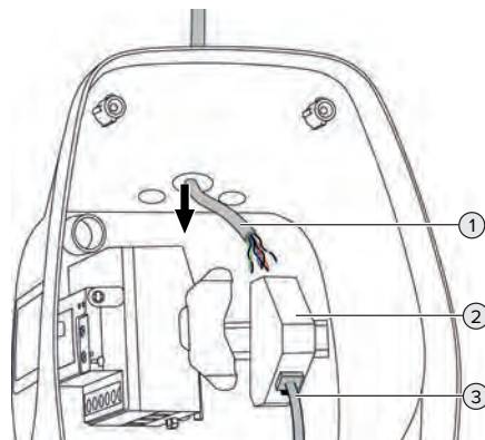
Afb. 14: Dataleiding aansluiten (voorbeeld)
