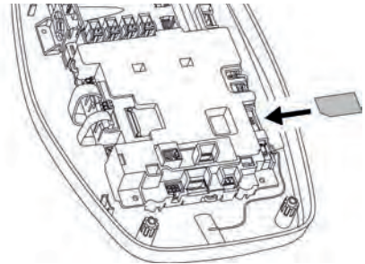
Abb. 11: SIM-Karte einsetzen
