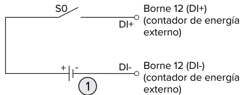
Fig. 17: Accionamiento mediante un relé acoplador y una alimentación de tensión adicional (en el estado de entrega)
