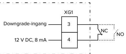
Afb. 16: Principeschema: aansluiting van een extern schakelcontact (standaardinstelling: NO)
