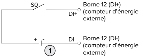
Fig. 17 : Activation par le biais d'un relais de couplage et d'une alimentation électrique supplémentaire (à l'état à la livraison)
