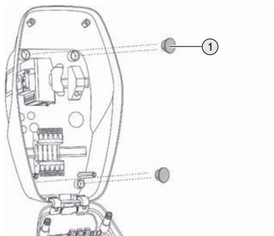
Afb. 7: Afsluitstoppen
