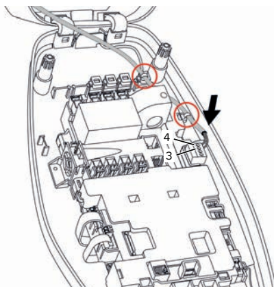
Afb. 15: Aansluiting downgrade-ingang
