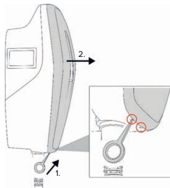
Fig. 4: Desmontar la cubierta frontal
