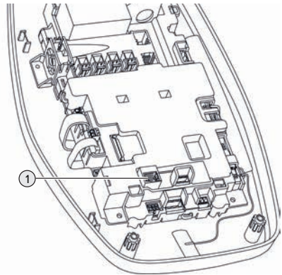
Abb. 13: Ethernet-Anschluss
