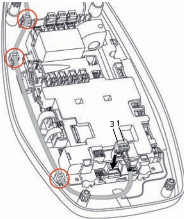
Abb. 9: Anschluss Arbeitsstromauslöser
