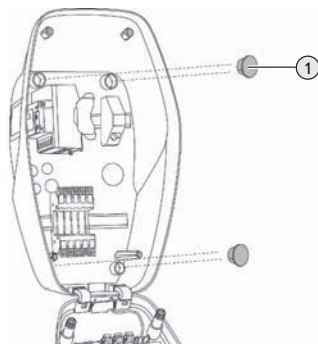
Abb. 7: Verschlussstopfen
