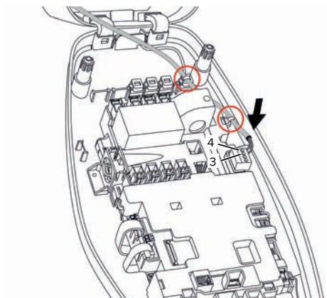
Fig. 15: Collegamento ingresso Downgrade
