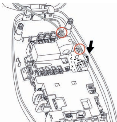
Fig. 15: Conexión entrada Downgrade
