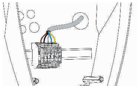
Abb. 8: Anschluss Spannungsversorgung
