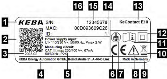
Abb. 4-4: Beispiel Typenschild
