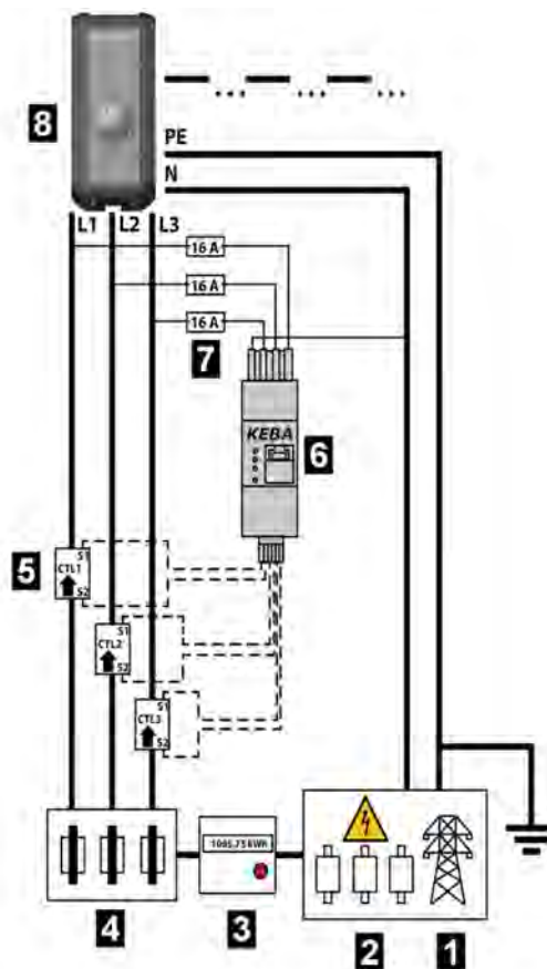
Abb. 7-6: Anschlussübersicht 3-phasig
