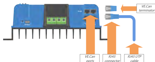
VE.Can-Anschluss, Stecker, Abschlusswiderstand und Kabel
