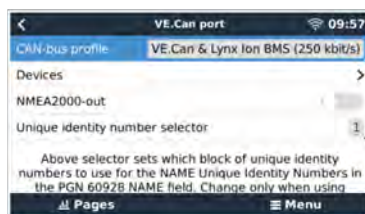
GX-Bildschirm mit Einstellung des CAN-Bus-Profiles
