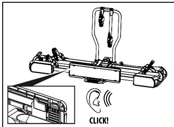
Bild 5: Kennzeichenhalter einrasten
