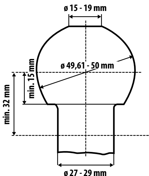
Bild 2: Dimensionen Kupplungskugel
