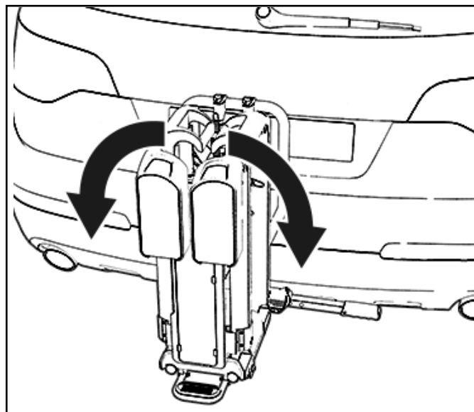
Figura 17: Svolgimento del portabici
