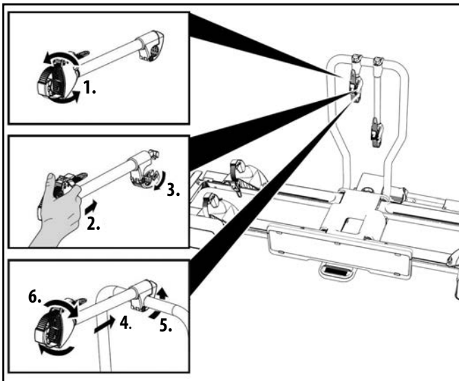
Bild 9: Montage Rahmenhalter
