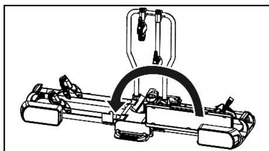
Bild 4: Kennzeichenhalter schwenken
