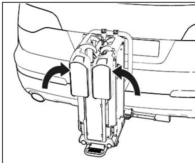
Bild 34: Zusammenklappen des Fahrradträgers
