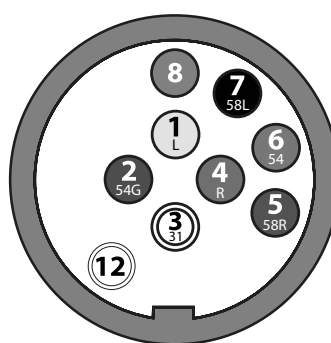
Stekker
