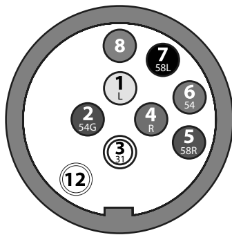
Connettore
