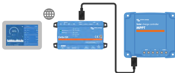
Verbindung der VictronConnect App über LAN oder das Internet (VRM Portal) mit einem GX-Gerät (z. B. einem Cerbo GX)
