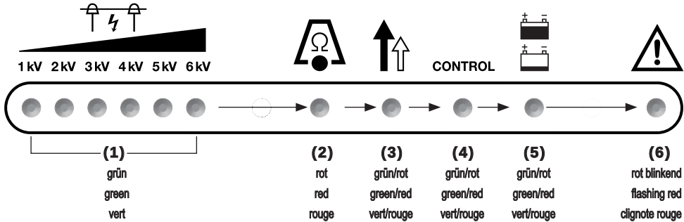
Fig. 3 / LED-Test
