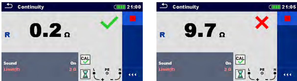
Abbildung 7.21: Beispiele für Ergebnisse der kontinuierlichen Durchgangsprüfung
