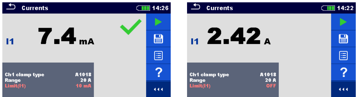
Abbildung 7.61: Beispiele für Ergebnisse der Strommessung
