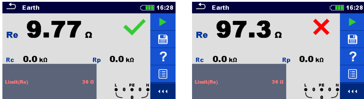
Abbildung 7.49: Beispiele für Ergebnisse der Erdungsmessung
