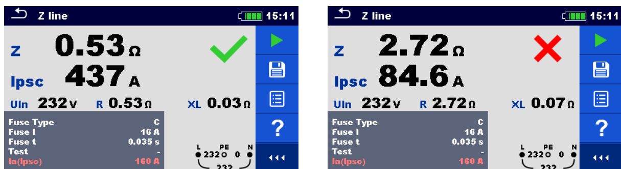
Abbildung 7.38: Beispiele für Ergebnisse der Leitungsimpedanzmessung
