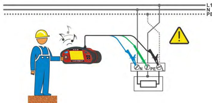
Abbildung 1.2: Vertauschte Leiter L und PE (Verwendung der 3-Leiter Prüfleitung)
