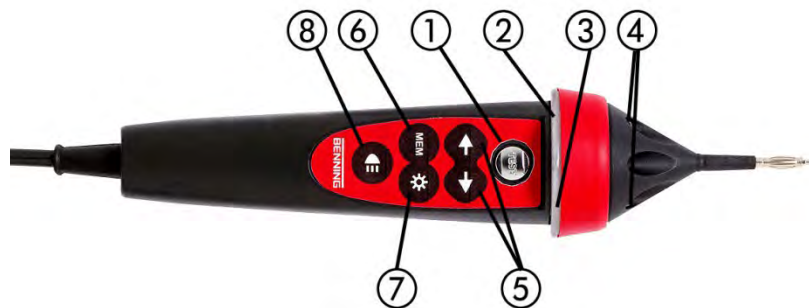
Abbildung A.2: Vorderseite der optionalen Commander-Prüfspitze (044155)
