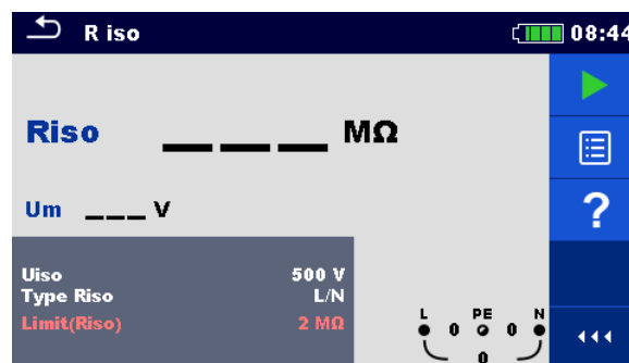
Abbildung 6.2: Startbildschirm einer Einzelprüfung, Beispiel für Isolationswiderstandsmessung
