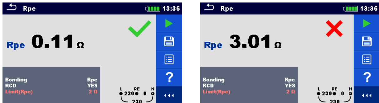
Abbildung 7.68 Beispiele für Ergebnisse der Schutzleiterwiderstandsmessung
