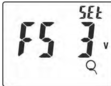
Abb. 5: Einstellung des Messbereiches der flexiblen Strommesszange
