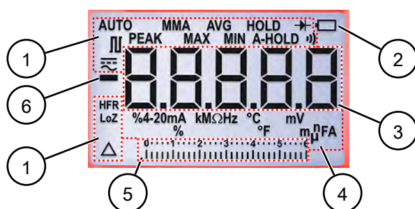
Abb. 8: Digitalanzeige
