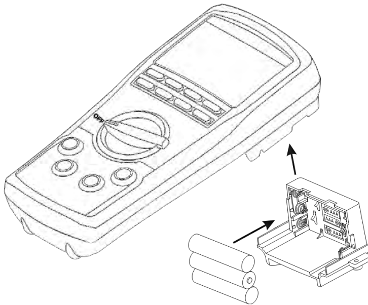
Abb. 16: Batteriewechsel (beispielhaft)
