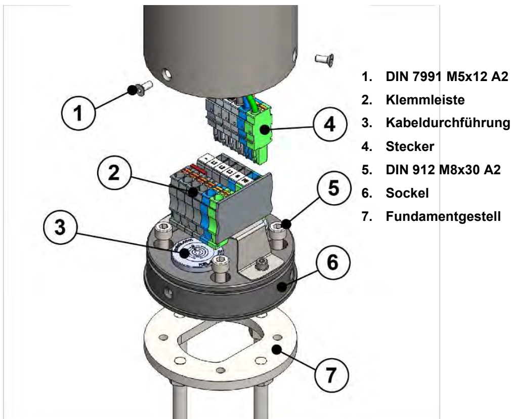
Montage in Kombination mit Fundamentgestell
