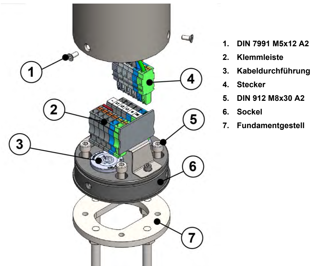
Montage in Kombination mit Fundamentgestell
